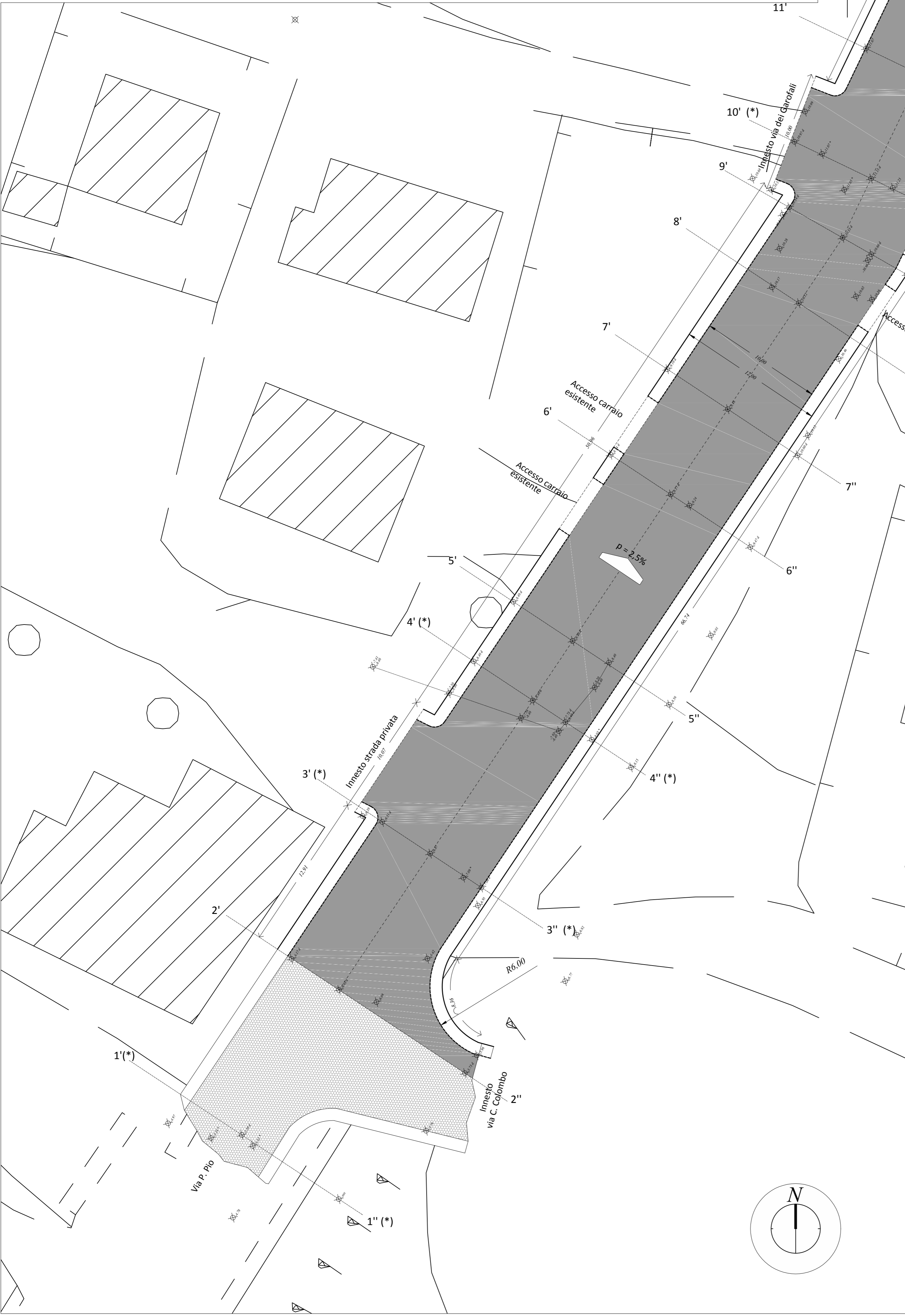
Planimetria di progetto scala 1:200
